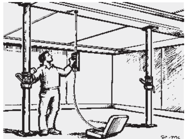
Anvendelse af en følerstang til nivellering af en loftforskalling (Regulering med en énhåndsspindel)
